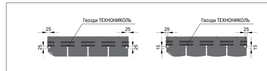
Рис. 3. Схема крепления фасадной плитки на 5 гвоздей
