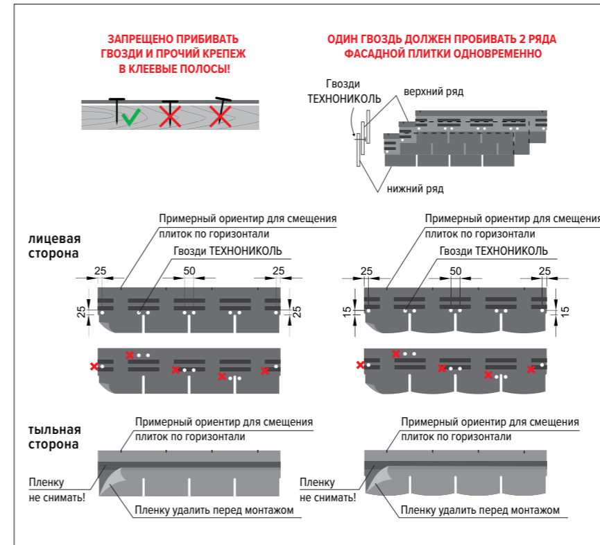
Рис. 2. Схема крепления фасадной плитки на 8 гвоздей
