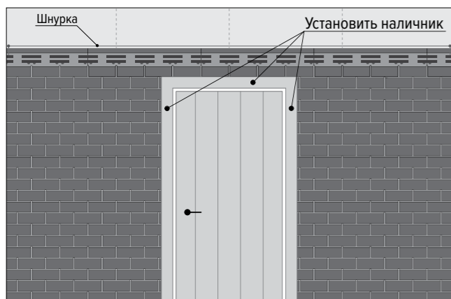
Рис. 12. Установка наличников
