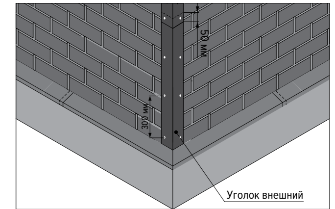
Рис. 9. Устройство внешних углов
