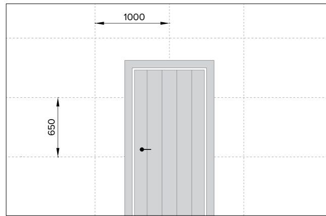
Рис. 4. Разметочные линии
