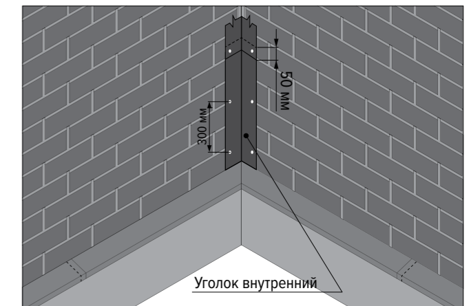
Рис. 10. Устройство внутренних углов
