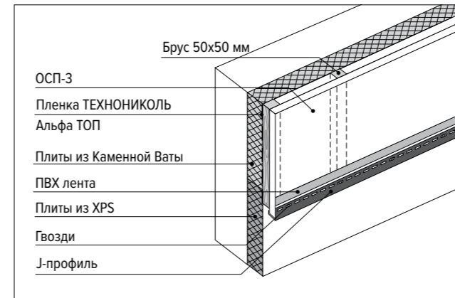
Рис. 6. Монтаж J-профиля
