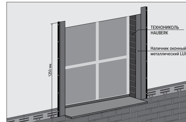
Рис. 20. Монтаж фасадной плитки вокруг оконных проемов
